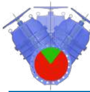
DN350 ➡ DN600
