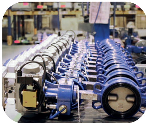
Absperrklappe mit doppelwirkendem pneumatischen Antrieb, Not-Handrad und Magnetventile
