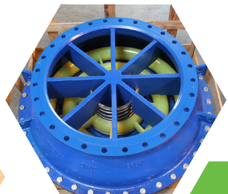
DN900
