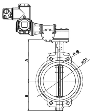
DN350 - DN600
