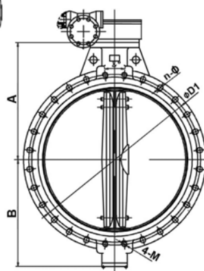
DN700 - DN1200
