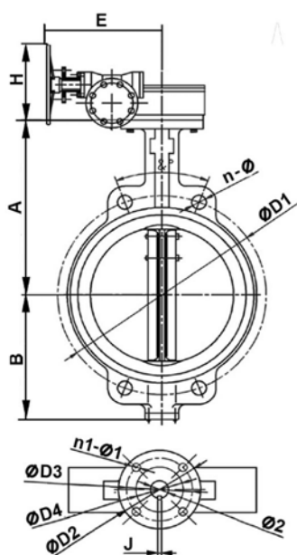
DN350 - DN600
