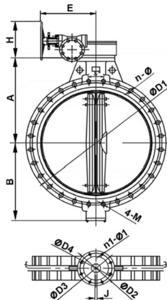
DN700 - DN1200
