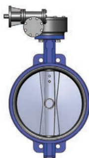
DN400-500
