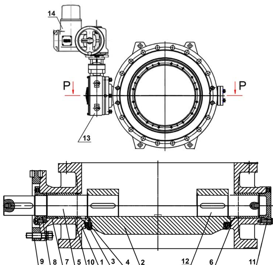
Вид Р-Р
