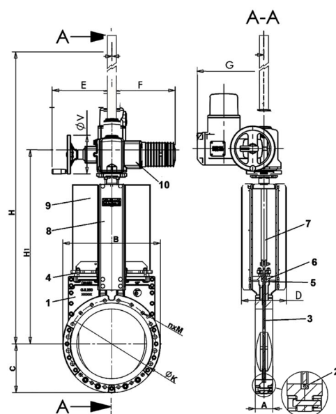
Ду450-600
