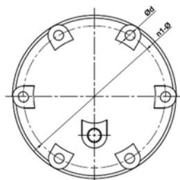
Vue A (DN125-300)
