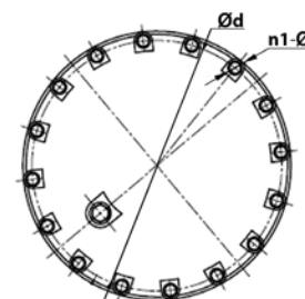
Vue A (DN350-400)
