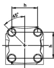
Vue A (DN15-32)
