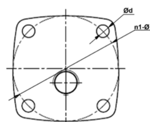
Vue A (DN50-80)
