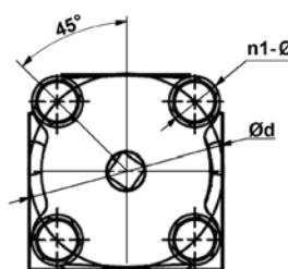
Vue A (DN40)
