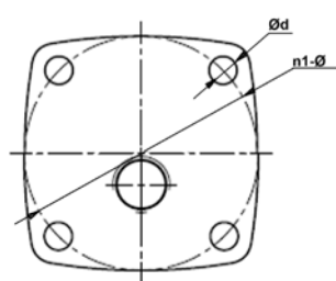
Vue A (DN100)
