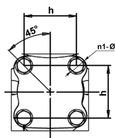
Вид А (Ду15-32)
