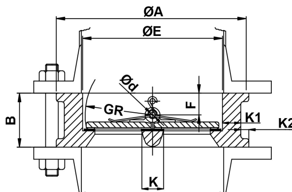
Вид A-A
