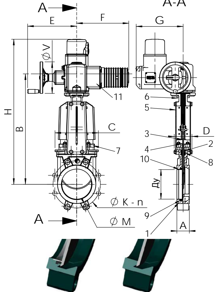
Стандартное уплотнение
