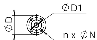
Embase normalisée suivant ISO 5211.
